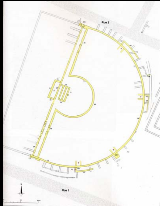
226. Le théâtre 2 (phase 4) état 1. Ech. 1/500.
