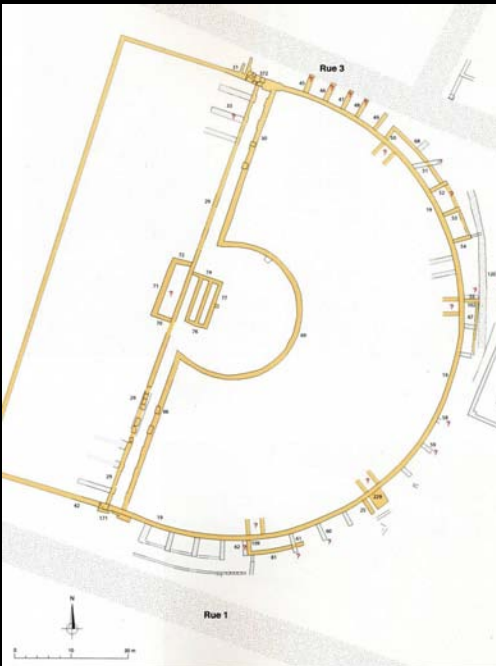
Fig. 230. Le théâtre 2 (phase 4) état 2. Ech. 1/500.
