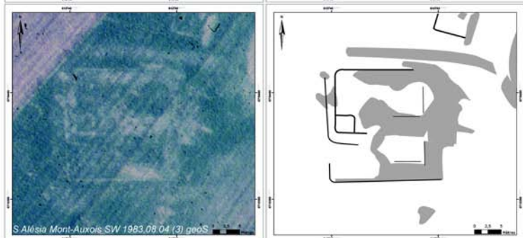
Extrait d'un cliché aérien de R. Goguet (1983) redressé : le temple d'en Surelot et interprétation technique
