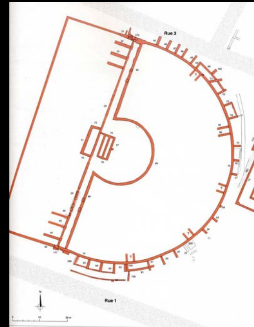
231. Le théâtre 2 (phase 4) état 3b. Ech. 1/500.
