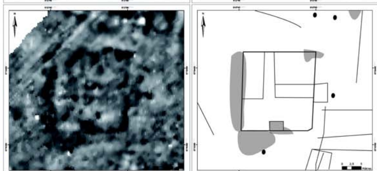
Extrait du relevé magnétique sur le temple d'en Surelot et interprétation technique
