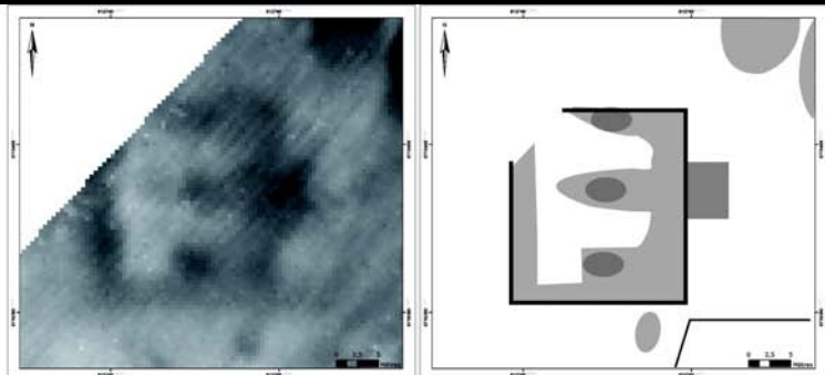
Extrait du relevé électrique sur le temple d'en Surelot et interprétation technique
