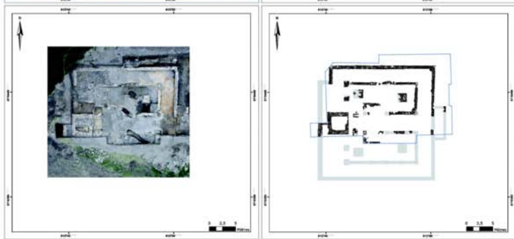
Extrait d'un cliché de la fouille du temple d'en Surelot (Cazanove & Osanna dir.), plan du bâtiment et relevé des structures fouillées
