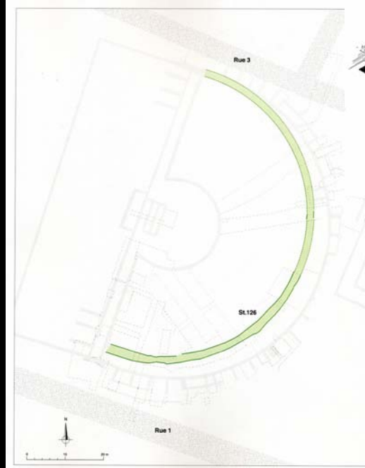
Fig. 225. La travée St. 126 de l'hypothétique théâtre 1 (phase 3). Ech. 1/500.
